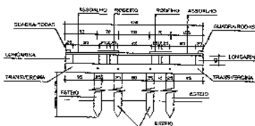
SEÇÃO TRANSVERSAL-ESC.1: 50
