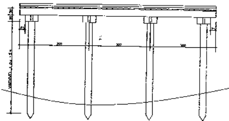
SEÇÃO LONGITUDINAL-ESC.1: 50
