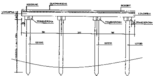
SEÇÃO LONGITUDINAL-ESC.1: 50
