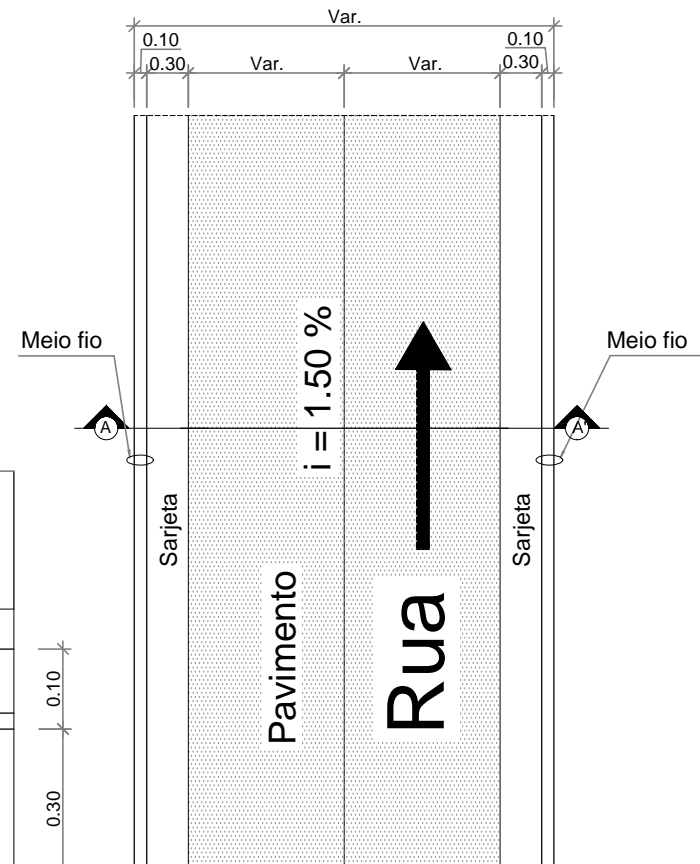
DETALHE PAVIMENTAÇÃO Esc.: 1/20
