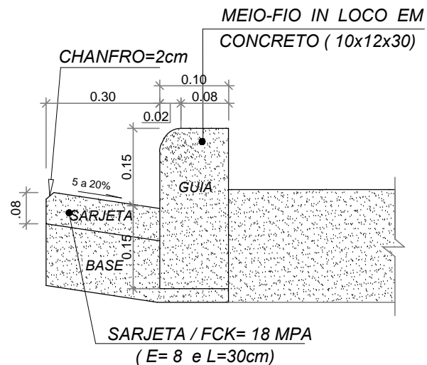
VISTA DE MEIO FIO E SARJETA S/ ESCALA
