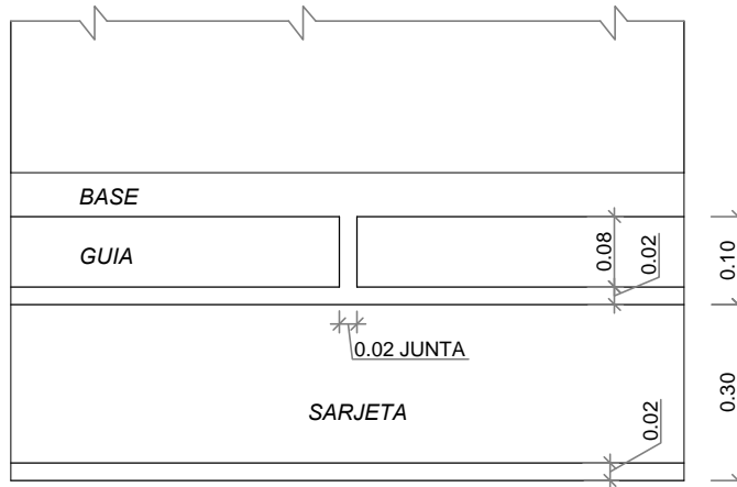
PLANTA BAIXA DE MEIO FIO E SARJETA S/ ESCALA
